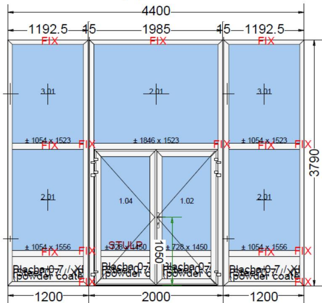
Poz.č. 9 Vonkajší pohľad dvere von otváravé
