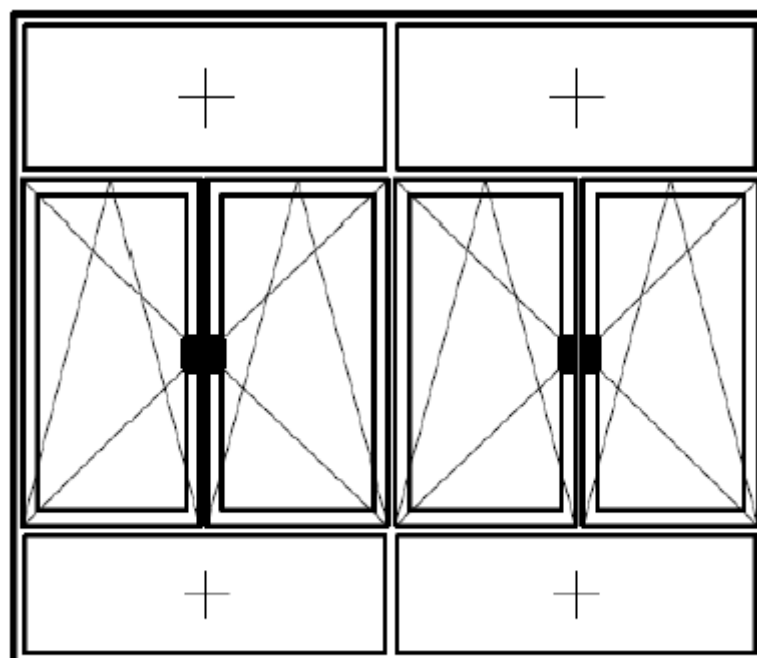
Poz.č. 8 Vnútorňý pohľad
